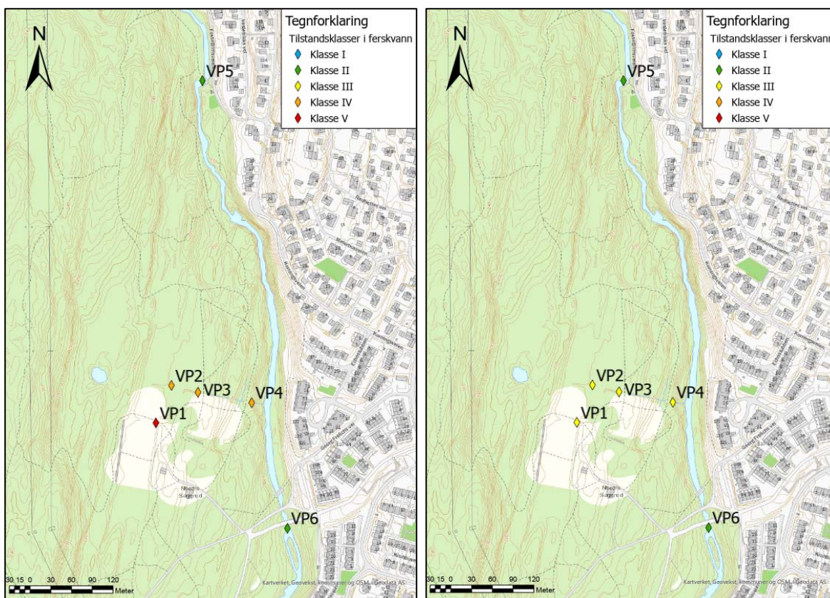
Figur 32. Plassering av vannprøvepunkter, og høyeste påviste tilstandsklasser i ferskvann iht. veileder M-608/2016. T.v. fra nedbørshendelsen 28. juni 2022 og t.h. fra tørrperioden 2. august 2022.
