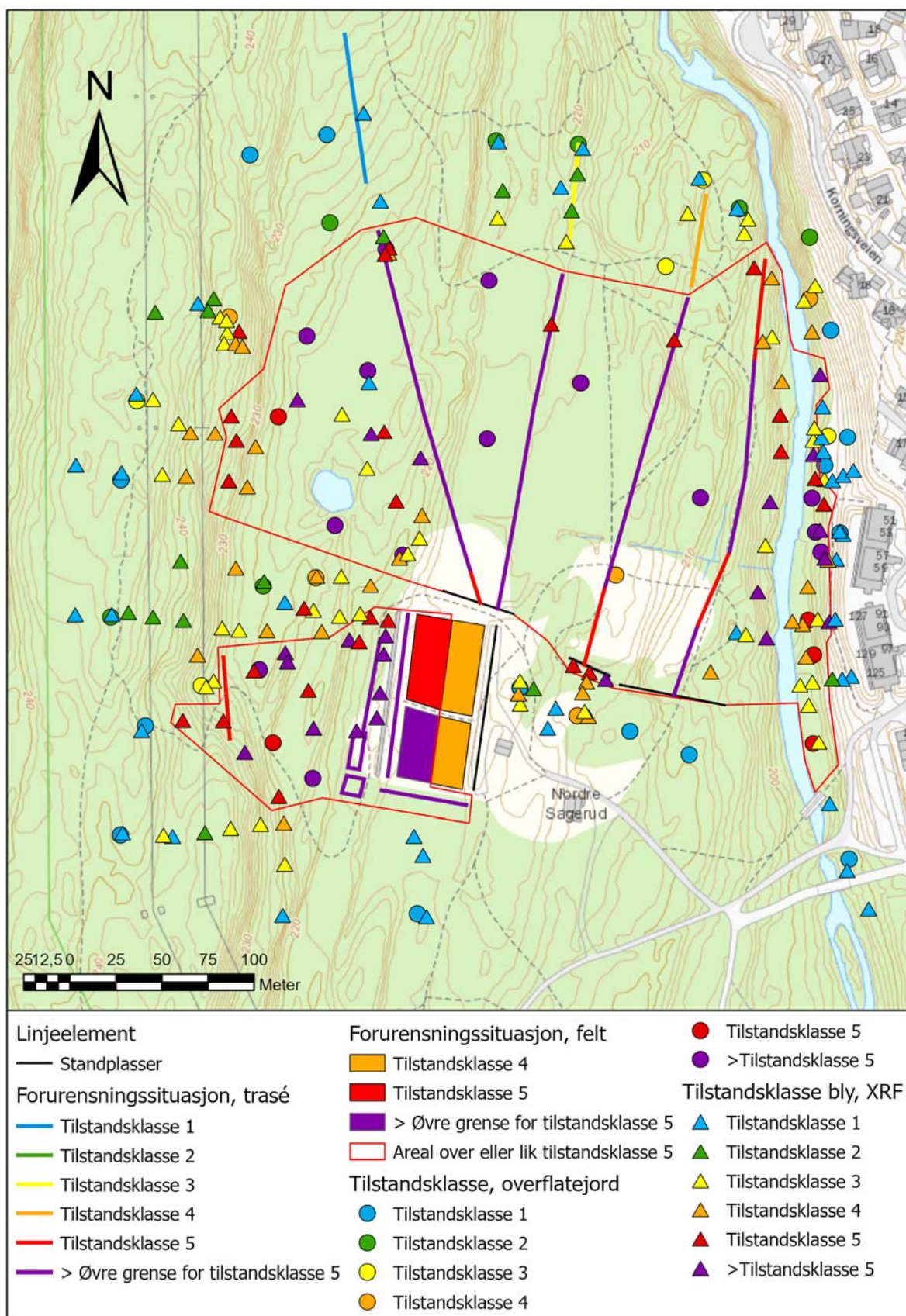
Figur 34. Samlet grunnforurensningssituasjon fra jordprøvetaking i 2021 og 2022 samt kartfestede XRF-målinger. Arealene med tilstandsklasse over eller lik klasse 5 og lengden på linjesegmentene mot nord er tilpasset nye resultater for området.
