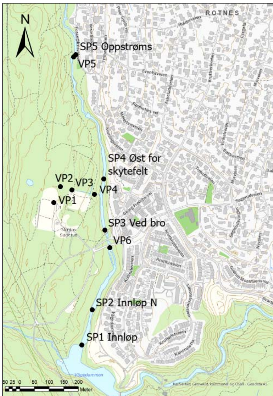
Figur 4. Oversikt over vann (VP)- og sedimentprøvene (SP). Vann- og sedimentprøvepunktene som ligger oppstrøms sammenfaller med hverandre.
