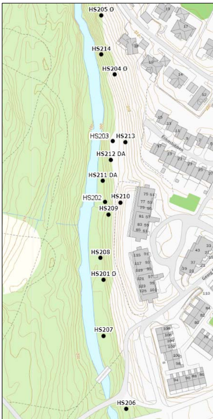
Figur 3. Prøvepunktene plassering øst for Ørfiskebekken. Punktene HS201 til HS205 ble tatt i august, 2022, mens HS206-HS214 ble tatt ut i den supplerende prøvetakingen i november 2022.
