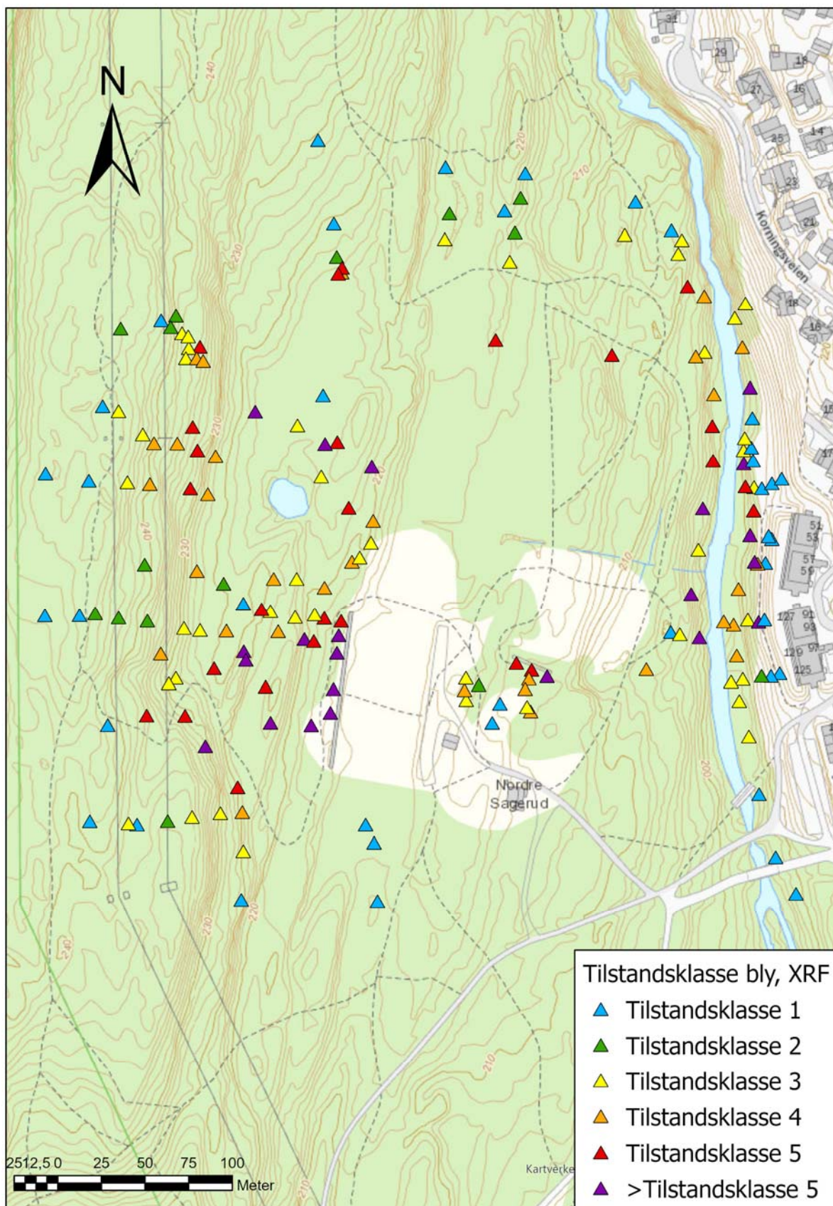
Figur 27. Forurensningsgraden for de kartfestede XRF-målingene fra den utvidede utredningen på Sagerud (august og november 2022), med høyeste påviste forurensning fargekodet iht. veileder for helsebaserte tilstandsklasser TA-2553/09.
