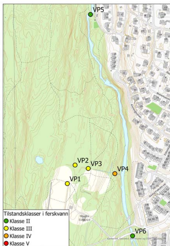
Figur 30. Plassering av vannprøvepunkter, og fargekodet iht. tilstandsklasser for bly i ferskvann fra veileder M-608/2016 i første utredning. Vannprøvene ble tatt i november 2021. Det er ikke registrert noe nedbør på nordre Sagerud i dagene før eller under prøvetakingsperioden (19.-25. november 2021).
