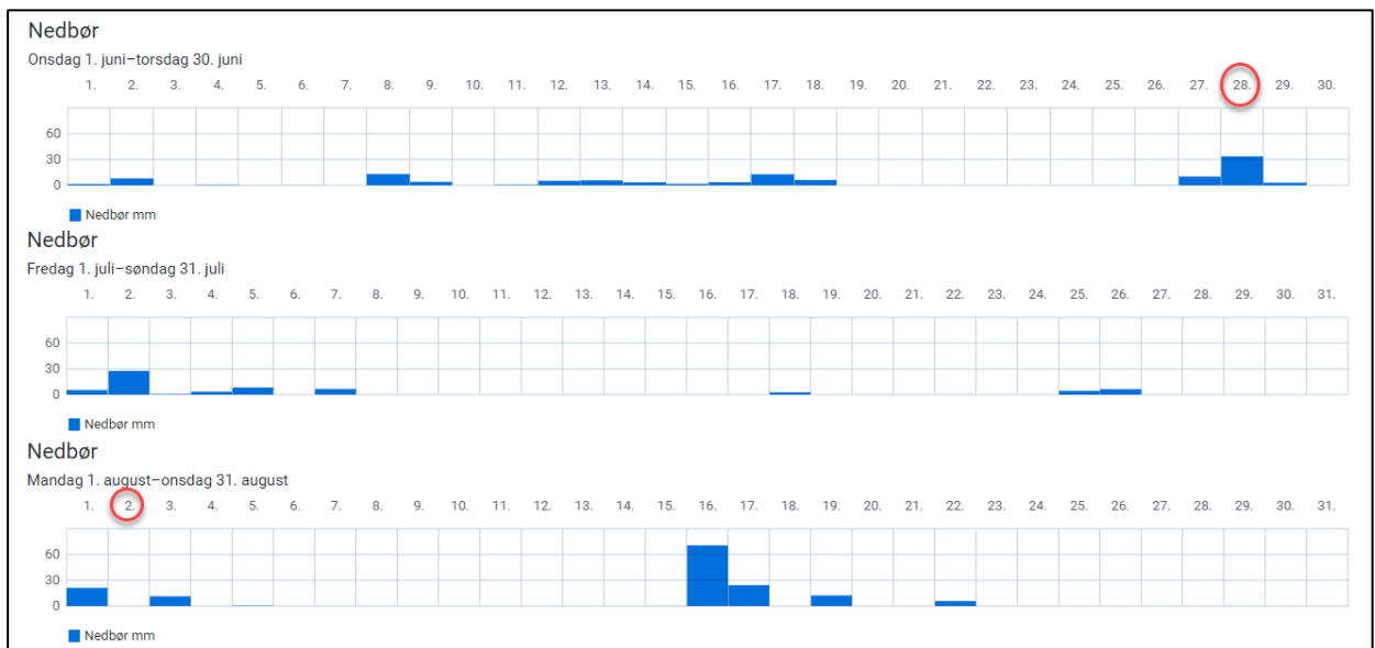
Figur 29. Nedbørsstatistikk fra nordre Sagerud viser at det var noe nedbør før og ilt. 28. juni, og relativt tørt en stund før 2. august, men med noe nedbør dagen før. Det er satt rød ring rundt de aktuelle prøvetaksdatoene. Kilde: yr.no.
