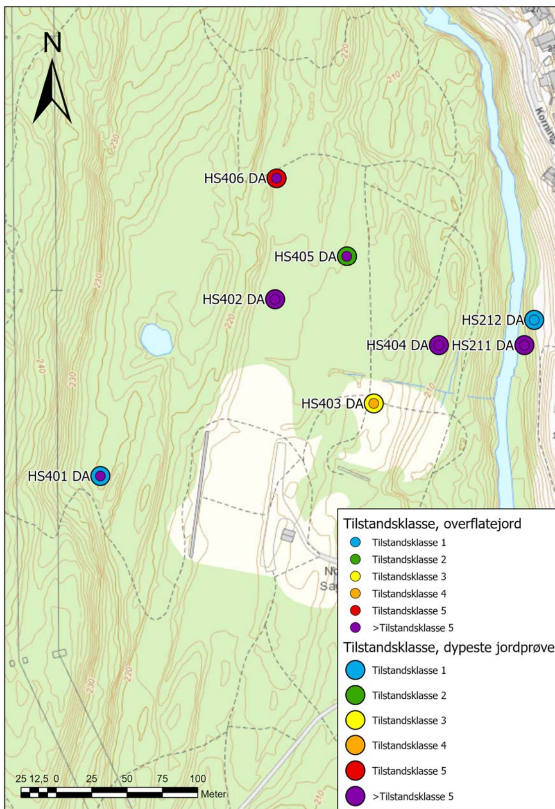
Figur 28. Forurensningsgraden fra prøvepunktene som hadde dypereliggende (under overflatejorda) prøver på Sagerud, med høyeste påviste forurensning fargekodet iht. veileder for helsebaserte tilstandsklasser TA-2553/09. Inkludert resultater fra prøvetaking august 2022 og november 2022, i 2021 ble det kun tatt prøver av toppjord.
