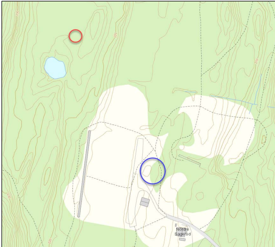
Figur 36. Omtrentlig plassering av observerte turdestinasjoner vest for Ørfiskebekken. Skogsområdet med bål plass er vist med rød sirkel og rasteplass/bål plass bak standplass er vist med blå sirkel.
