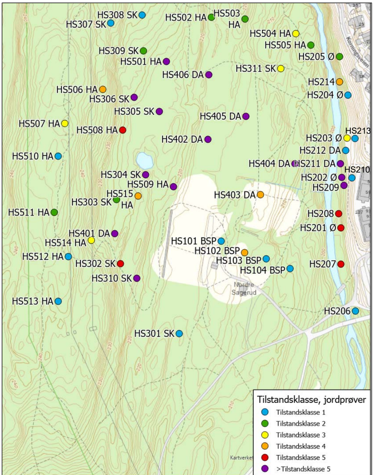
Figur 26. Forurensningsgraden for jordprøvene fra den supplerende utredningen på Sagerud fra august og november 2022 med høyeste påviste forurensning fargekodet iht. veileder for helsebaserte tilstandsklasser TA-2553/09. Resultater fra kartlegging i 2021 finnes i rapport 10229610-01-RIGm-RAP-001 [3].
