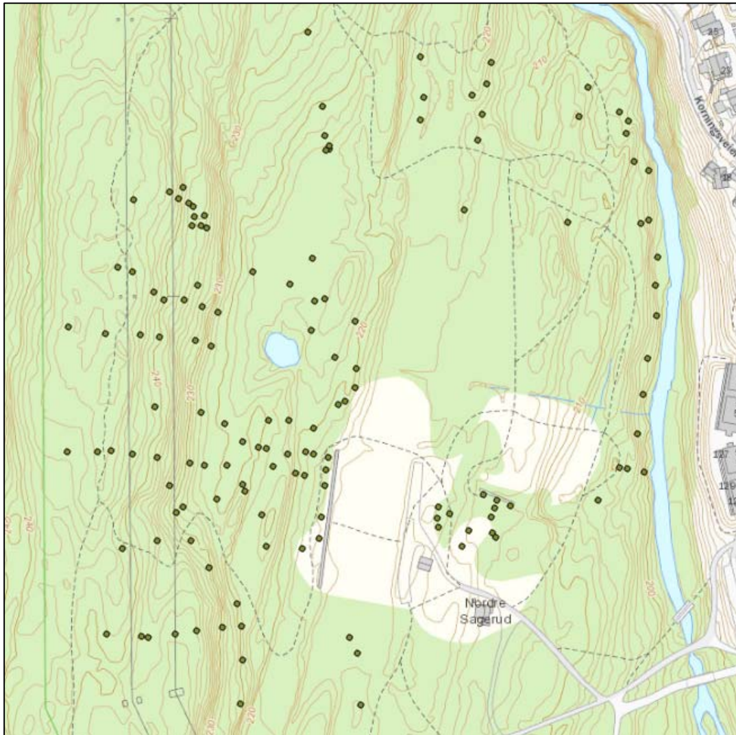
Figur 5. Plasseringen til XRF-målinger (kun august 2022) som ble målt inn med GPS og registrert. Plassering av supplerende målinger øst for Ørfiskebekken i november 2022 vises i Figur 27.
