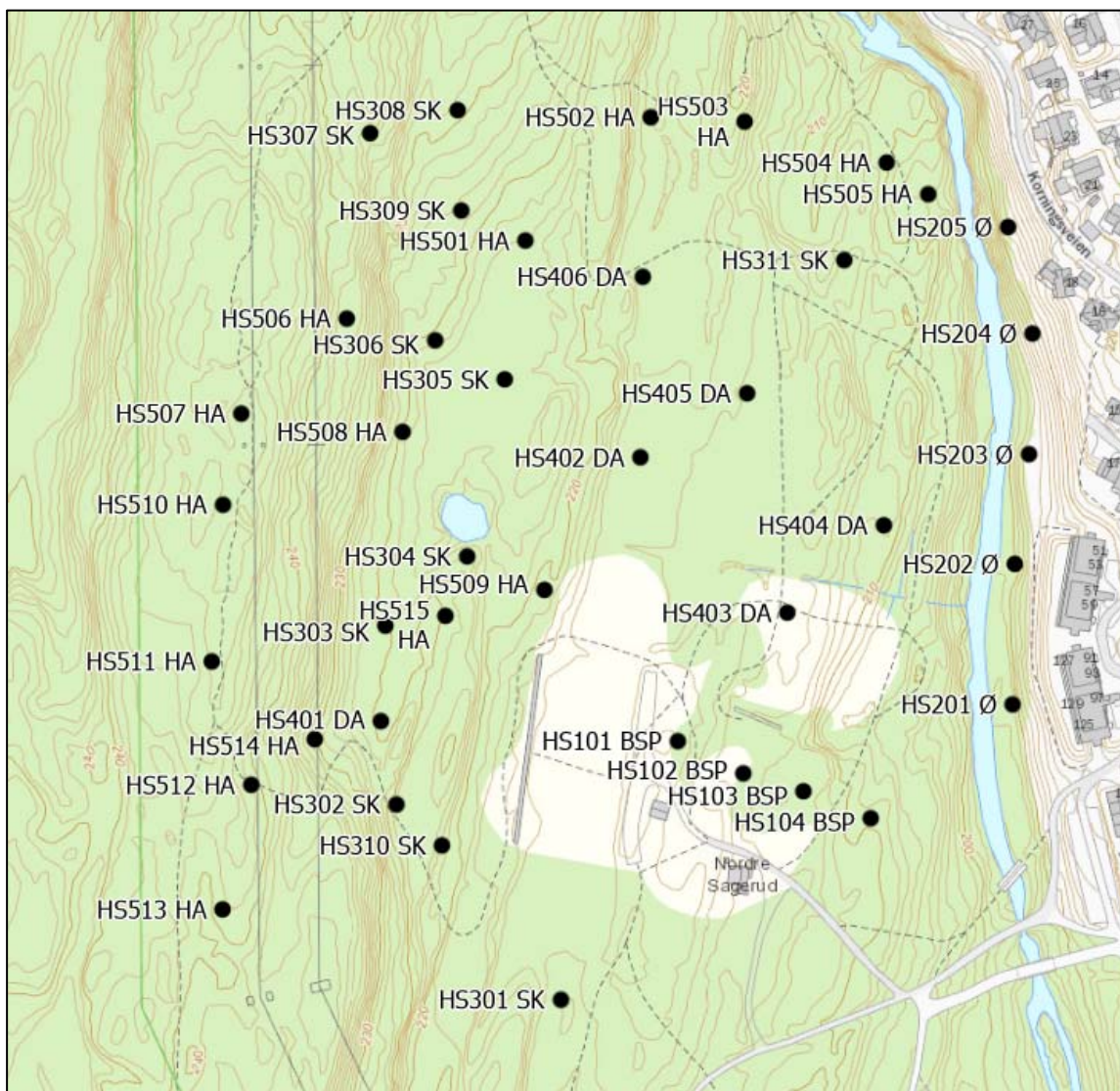
Figur 1. Utført prøvetaking av jordprøver i august 2022 (bakgrunnsprøvene fra nordre Sagerud er utenfor utsnittet, se figur 2 for plassering). Prøvepunktene er gitt ulikt suffiks: BSP = Bak standplass, Ø = Øst (for Ørfiskebekken), SK = Situasjonsskart, DA = Dybdeavgrensning, HA = Horisontalavgrensning. Prefiks HS = håndskovling, og hvert prøvenummer 101, 102, 201 ... osv. er et unikt prøvenavn. Prøvetaking fra 2021 er vist i [3], mens prøver tatt i november 2022 (punktene HS206-HS214) er vist i Figur 3.
