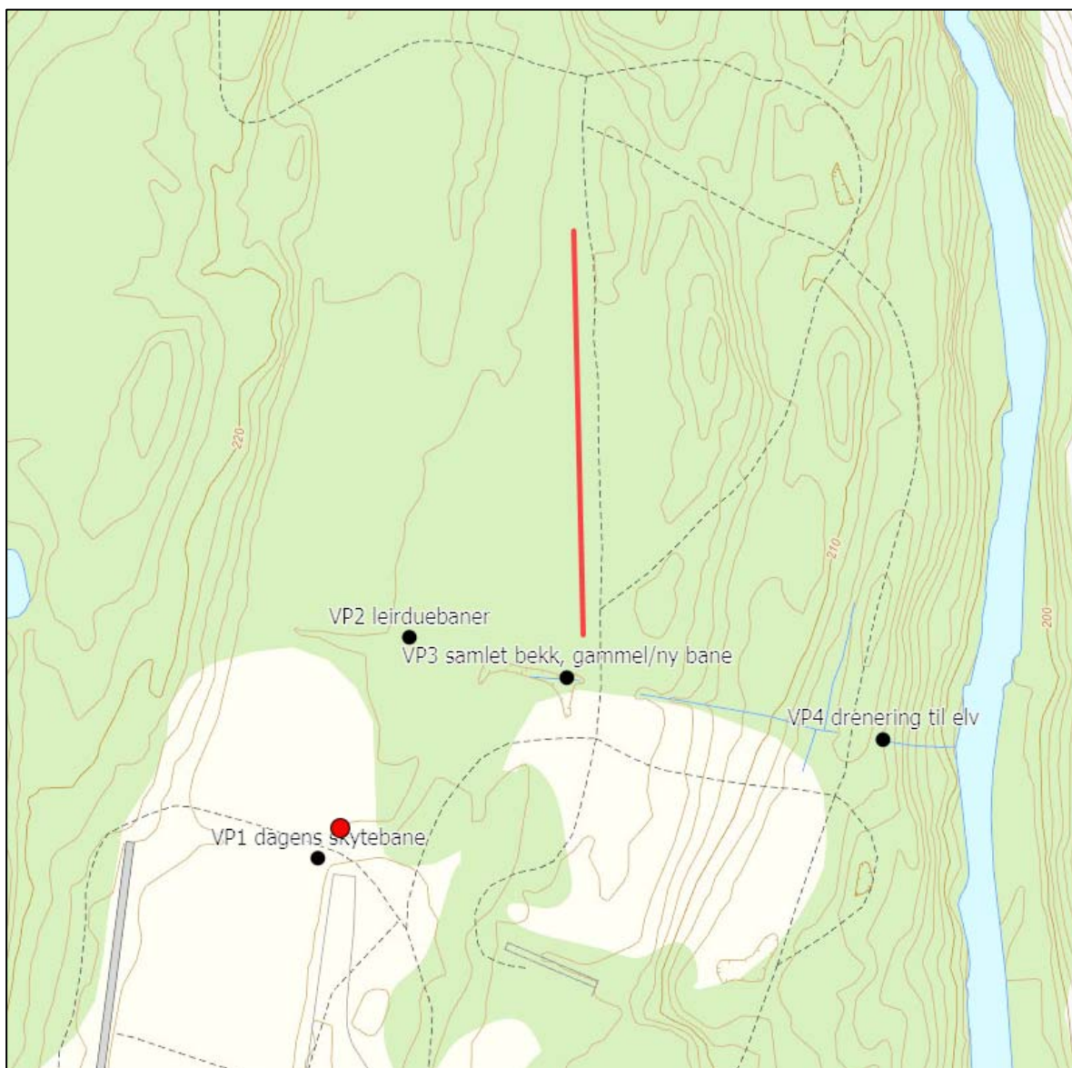
Figur 20. Linja markerer omtrentlig plassering av en nord-sørgående grøft som fører vann inn til grøftesystemet ved nedbør. Rødt punkt viser ny plassering av vannprøvepunkt 1.
