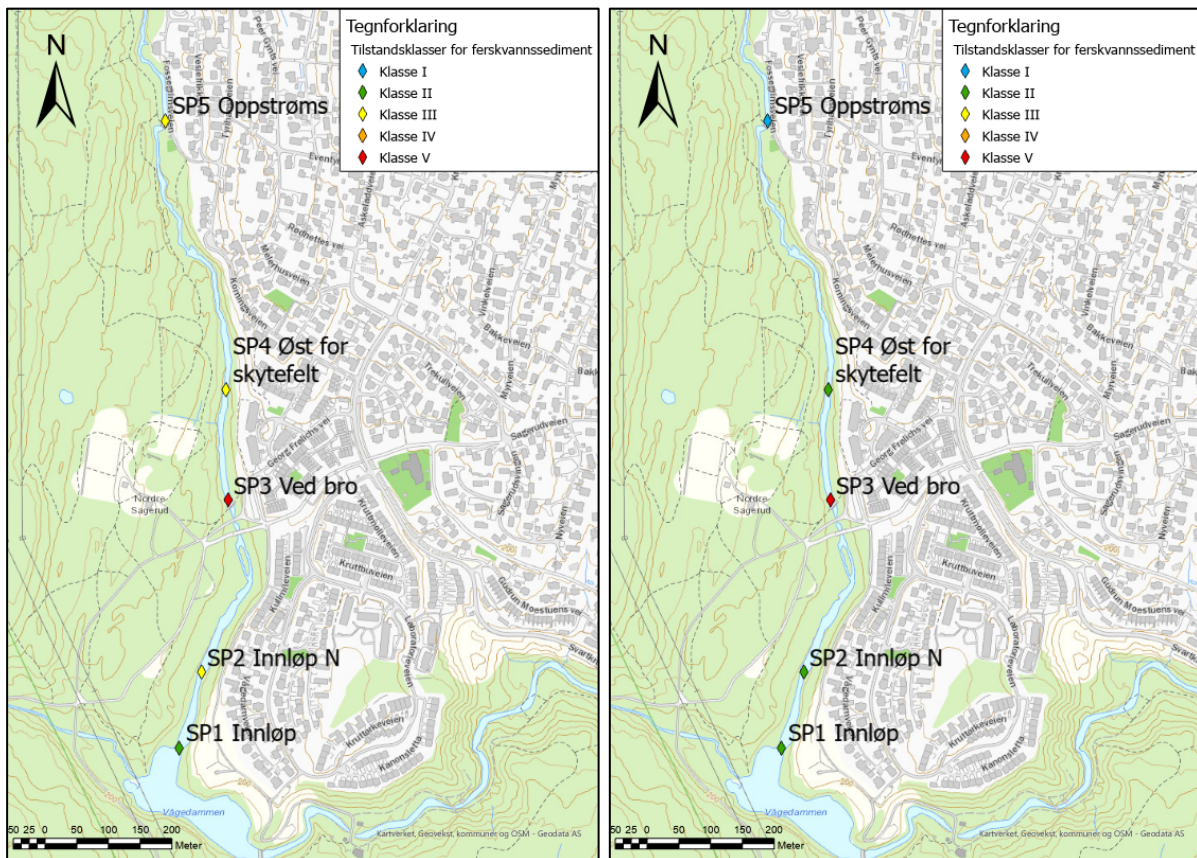
Figur 33. Plassering av prøvepunktene for sediment fargekodet iht. tilstandsklasser for ferskvannssediment iht. M608. T.v. er høyeste påviste tilstandsklasser for ferskvannssediment uavhengig av parameter, og t.h. er høyeste påviste tilstandsklasse for parametere forbundet med skyteaktiviteten på Sagerud (her er det bly og PAH som har gitt utslag over klasse I).
