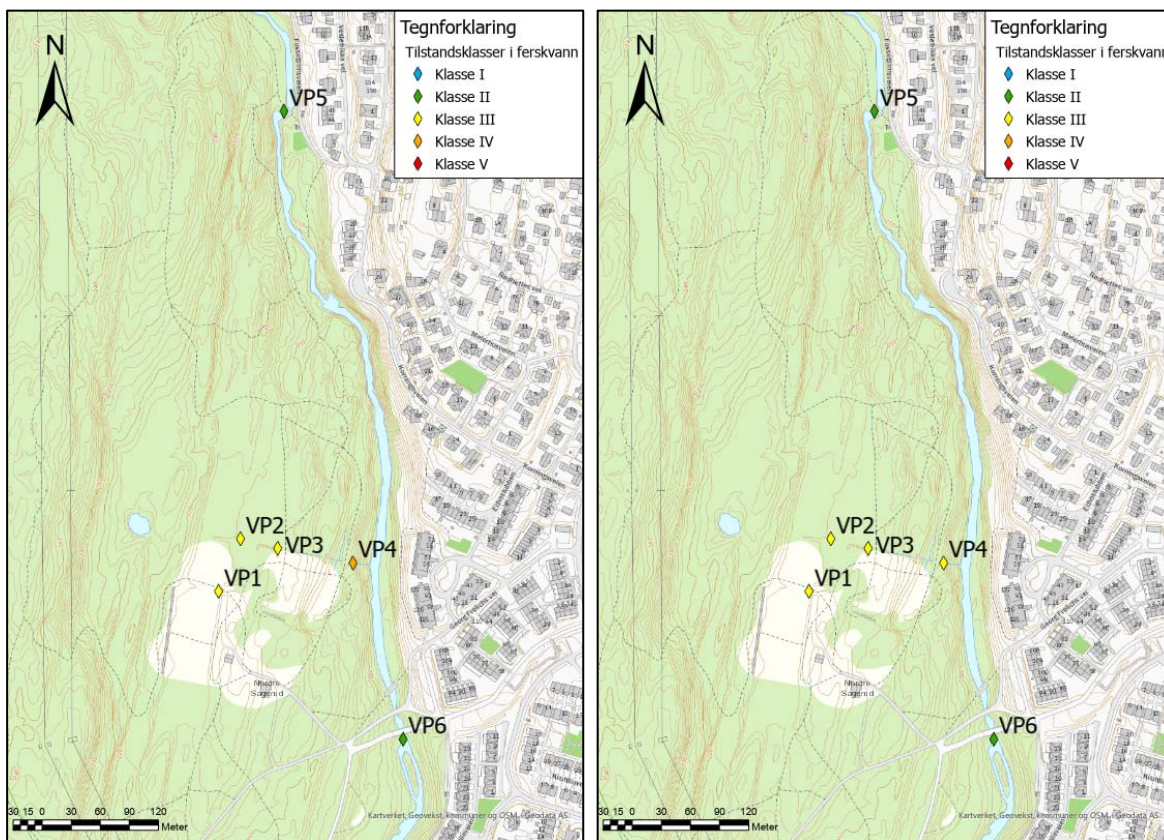
Figur 31. Plassering av vannprøvepunkter og tilstandsklasser for bly i ferskvann iht. veileder M-608/2016. T.v. fra nedbørshendelsen 28. juni 2022 og t.h. fra tørrperioden 2. august 2022.
